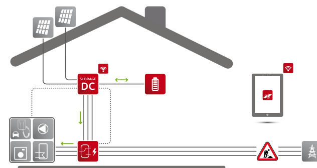
DC-SPEICHERSYSTEM MIT ERSATZSTROM RCT POWER STORAGE DC RCT POWER BATTERY RCT POWER SWITCH
