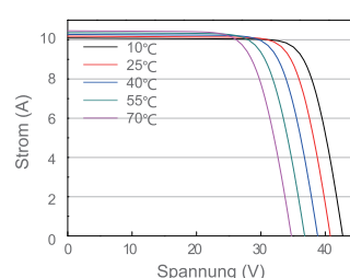
Strom/Spannungskurve JAM60S09-320/PR
