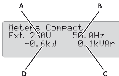
Abbildung 17: Übersicht des Menüs Meters Compact für den Generator oder das Ersatzstromnetz
