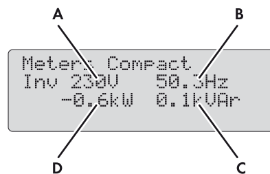
Abbildung 16: Übersicht des Menüs Meters Compact für die AC-Messwerte des Wechselrichters Sunny Island
