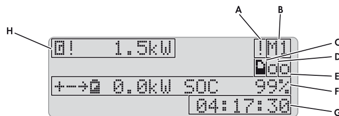
Abbildung 5: Energieflüsse und Statusmeldungen des Sunny Island
