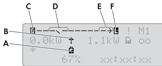
Abbildung 7: Grafische Darstellung der Energieflüsse im Standardmodus (Beispiel)
