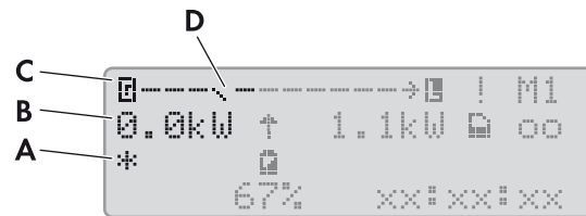
Abbildung 10: Status der externen Energiequelle im Standardmodus (Beispiel)
