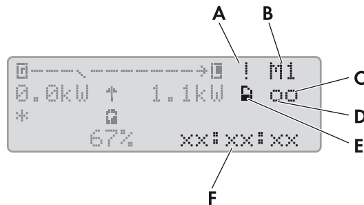
Abbildung 8: Status des Wechselrichters Sunny Island (Beispiel)
