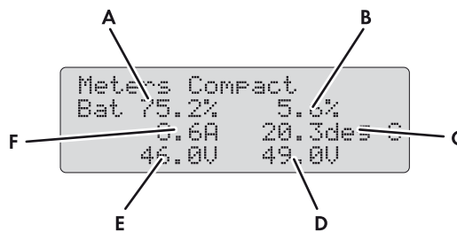
Abbildung 15: Übersicht des Menüs Meters Compact für die Batterie
