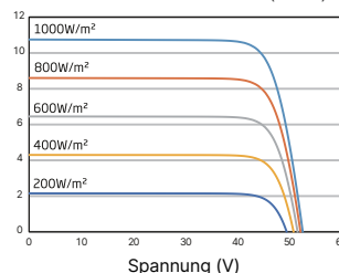
I-V-Kurven des PV-Moduls (445W)
