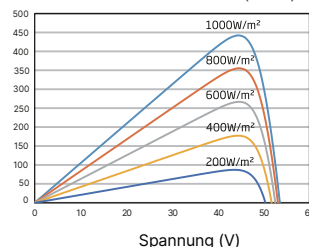
P-V-Kurven des PV-Moduls (445W)
