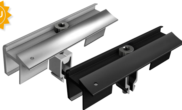
Endklemmen ohne Erdungspin für Rahmenhöhe 28 mm – 45 mm
