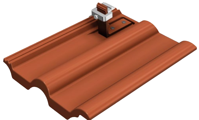
D-Platte passend für Frankfurter Pfanne RAL 8004 Kupferbraun (Ziegelrot) Art.-Nr. 11550-00
