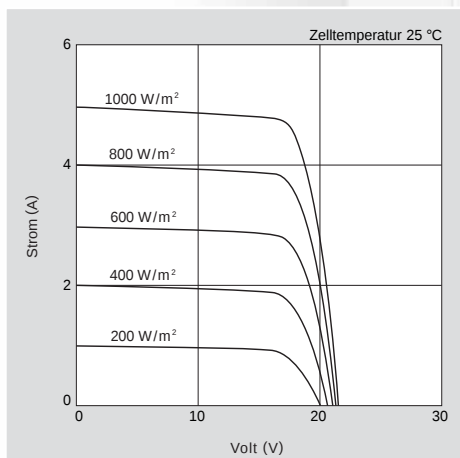
Strom-Spannungskennlinie des Moduls KC80-02 bei verschiedener Einstrahlung.
