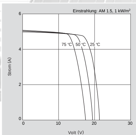
Strom-Spannungskennlinie des Moduls KC80-02 bei verschiedenen Zelltemperaturen.
